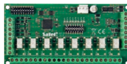
INT-O ekspander wyjść
