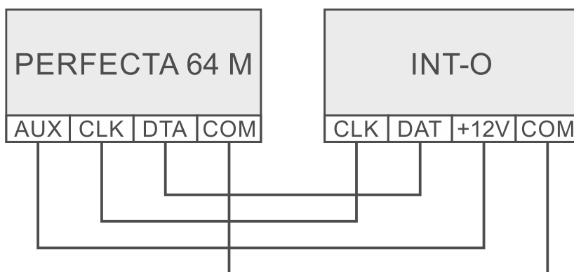
Rys. 10. Podłączenia ekspandera INT-O do centrali.
