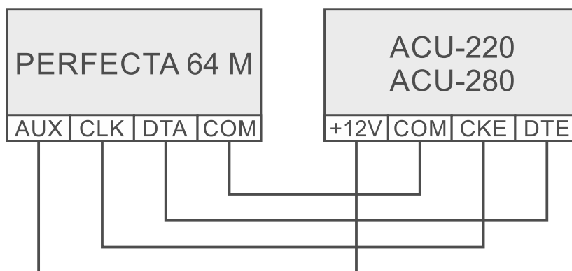
Rys. 7. Podłączenie kontrolera ACU-220 / ACU-280 do centrali.
