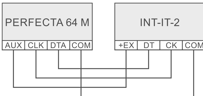
Rys. 11. Podłączenie modułu INT-IT-2 do centrali.
