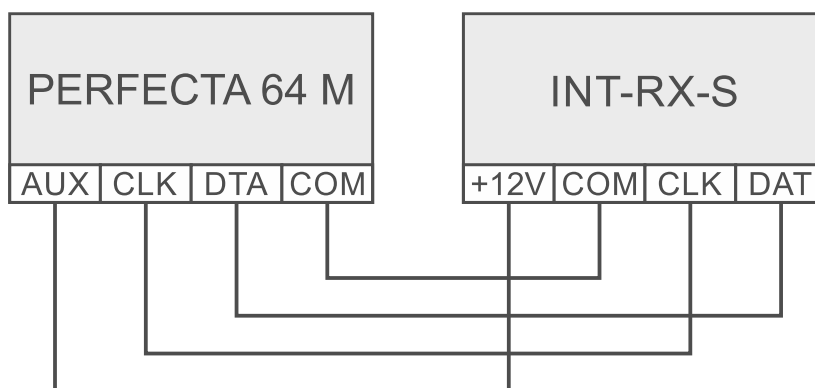
Rys. 8. Podłączenie ekspandera INT-RX-S do centrali.
